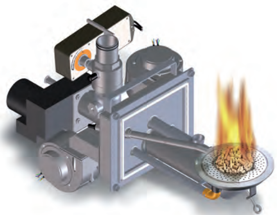
Pelletti Hightech im Detail: die Unterschubfeuerung mit der Verbrennungsretorte aus hochlegiertem Edelstahl.
